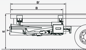
MOTRICE - PIANALE 1 RIPIEGAMENTO
