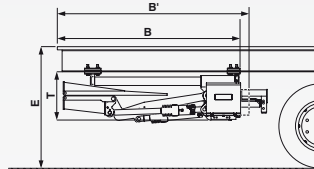
SEMIRIMORCHIO - PIANALE 1 RIPIEGAMENTO
